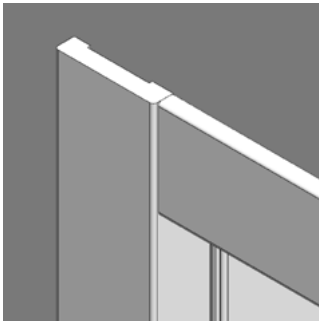
vodorovná obložková lišta 12 mm svislá obložková lišta 16 mm
