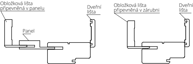
pro dveře CERBER PLUS
