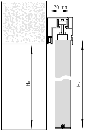
DĚLKY KRYCÍCH LIŠT POSUV. SYSTÉMU PREMIUM
