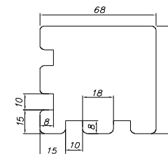
Úhlová spojka 90°
