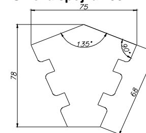
Úhlová spojka 135°
